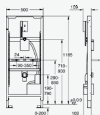
38 511 Rapid SL Urinoir-element Voor radarelektronica Zonder wandbevestiging
