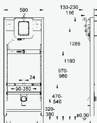
38 521 Rapid SL Urinoir-element Infrarood bediening Met wandbevestiging
