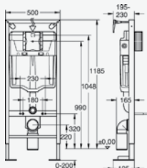
38 584 Rapid SL WC-element Vrijstaand, met wandbevestiging
